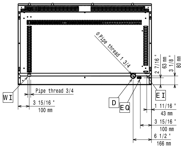
Felülnézet
